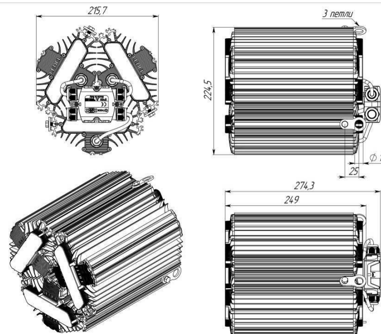
Рисунок 1 Светильник «L-lego 165». Подвесное крепление
