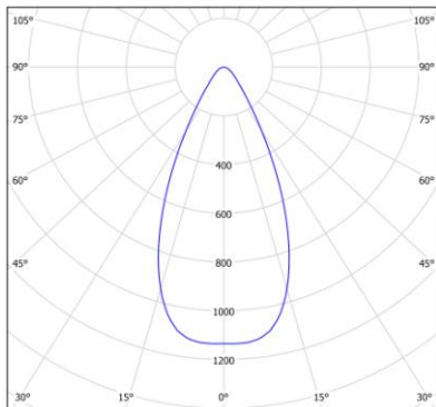
Исполнение «K12»
