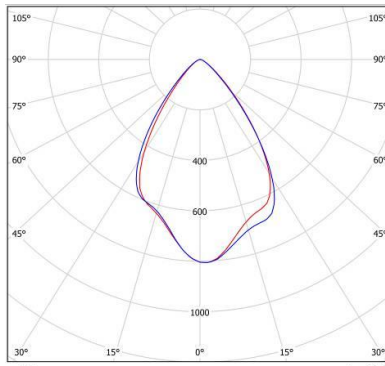
Исполнение «Г33»
