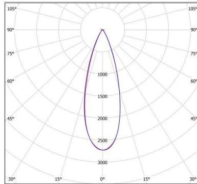
Исполнение «Г33»
