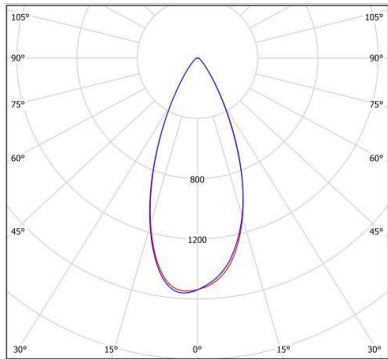
Исполнение «K12»
