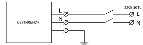
Рисунок 2 Схема подключения светильника ВОЗМОЖНЫЕ НЕИСПРАВНОСТИ И МЕТОДЫ ИХ УСТРАНЕНИЯ
